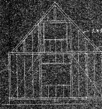
东面图
