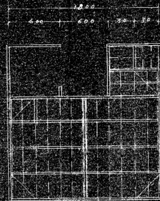
后屋平面图
