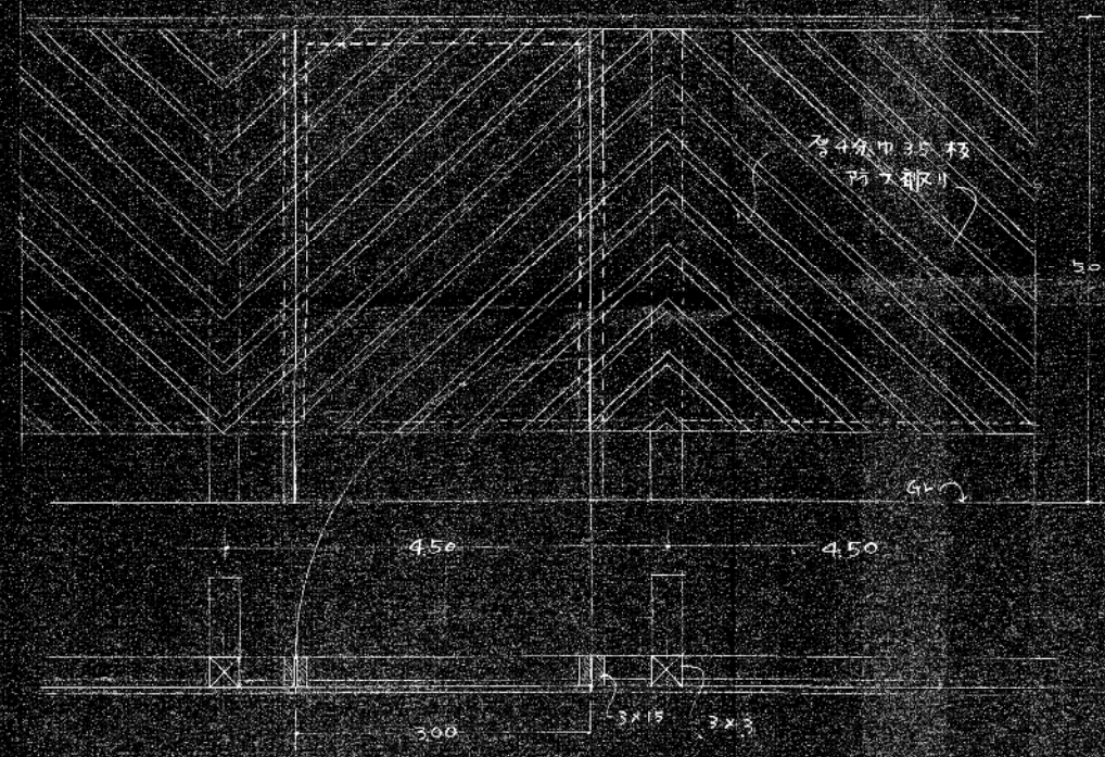
外廻板及ククリ詳細 (A 部)
